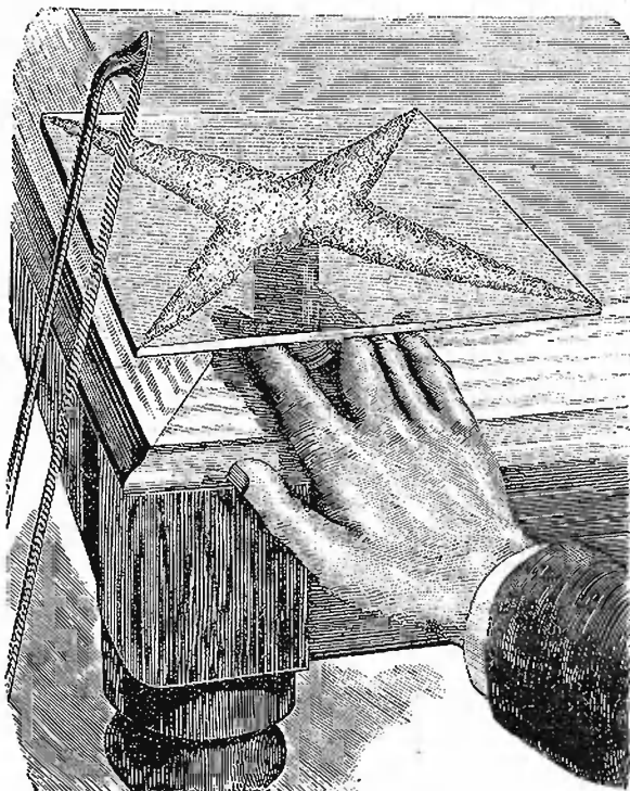
Фигуры, образующіяся изъ песка при сотрясеніи пластинки.
