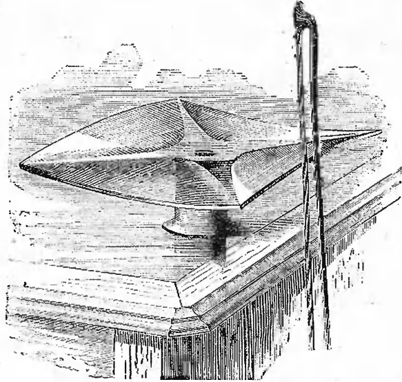
Узлы и петли, образующіяся изъ песка при сотрясеніи пластинки.
