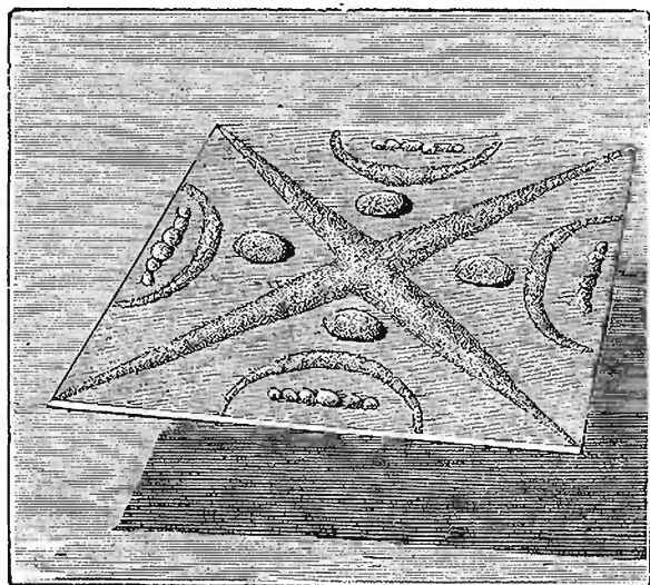
Фигуры, образующіяся изъ песка и плауноваго порошка при сотрясеніи пластинки.
